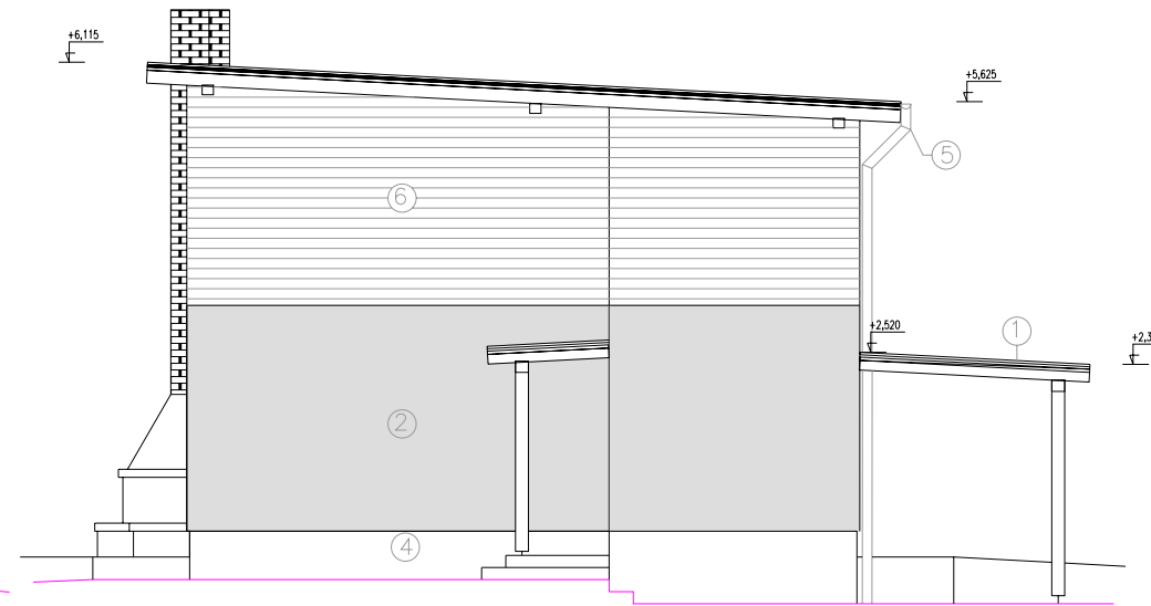
P?DORYS V?CHODN? :
