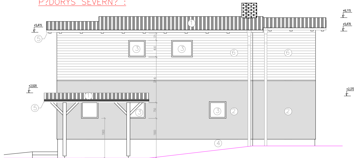
P?DORYS SEVERN? :
